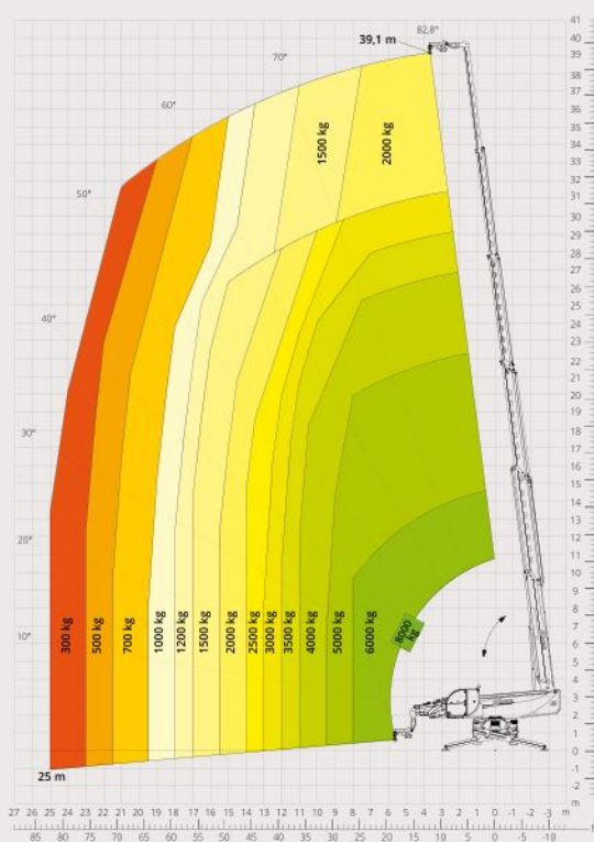
Diagram draagvermogens met HAAK 8.000 kg - M1
