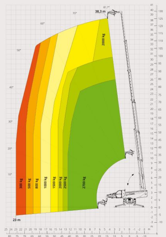
Diagram draagvermogens met GIEK MET LIER 2.700 kg
