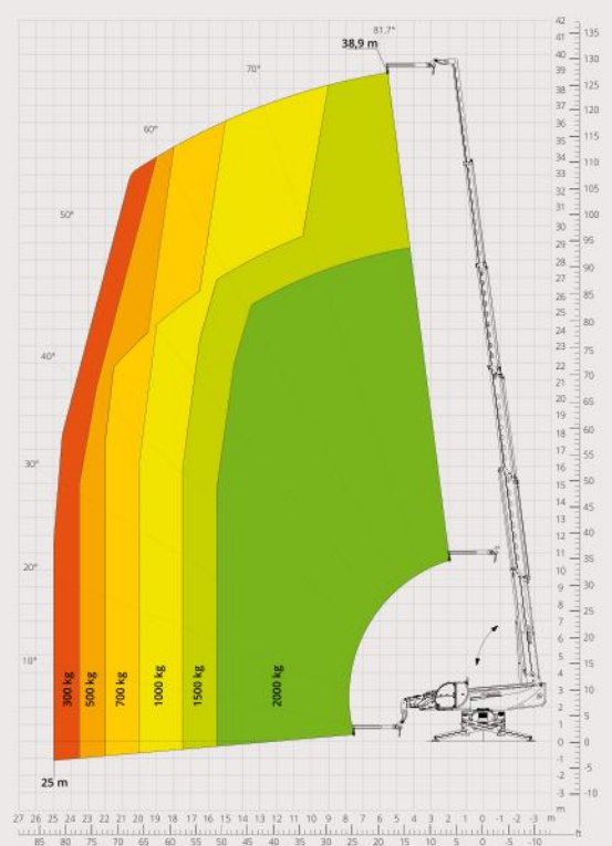
Diagram draagvermogens met GIEK 2.000 kg
