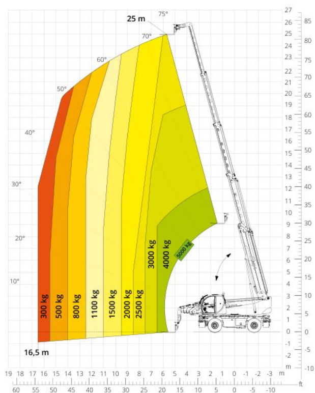
Diagram draagvermogens VOORZIJD OP BANDEN ATT - 03 - 007
