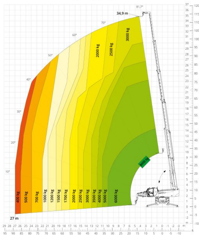
Diagram draagvermogens met UITGESCHOVEN STEMPELS 360° - M1 ATT - 03 - 007
