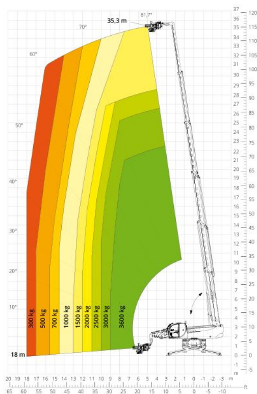
Diagram draagvermogens met VELKOP ATT - 08 - 001
