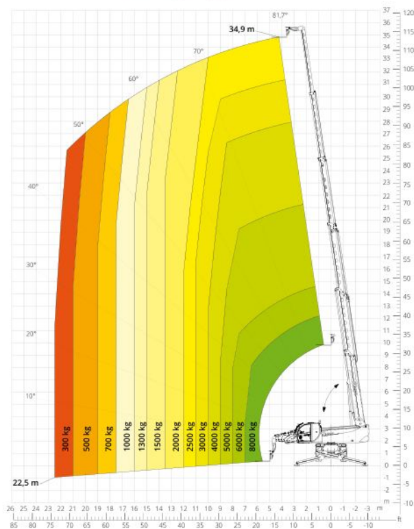
Diagram draagvermogens met UITGESCHOVEN STEMPELS 360° - M2 ATT - 03 - 007
