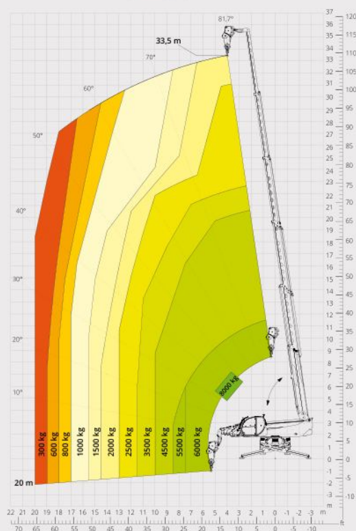
Diagram draagvermogens met LIER 8.000 kg - M1
