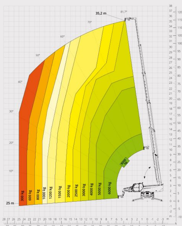
Diagram draagvermogens met HAAK 8.000 kg - M1
