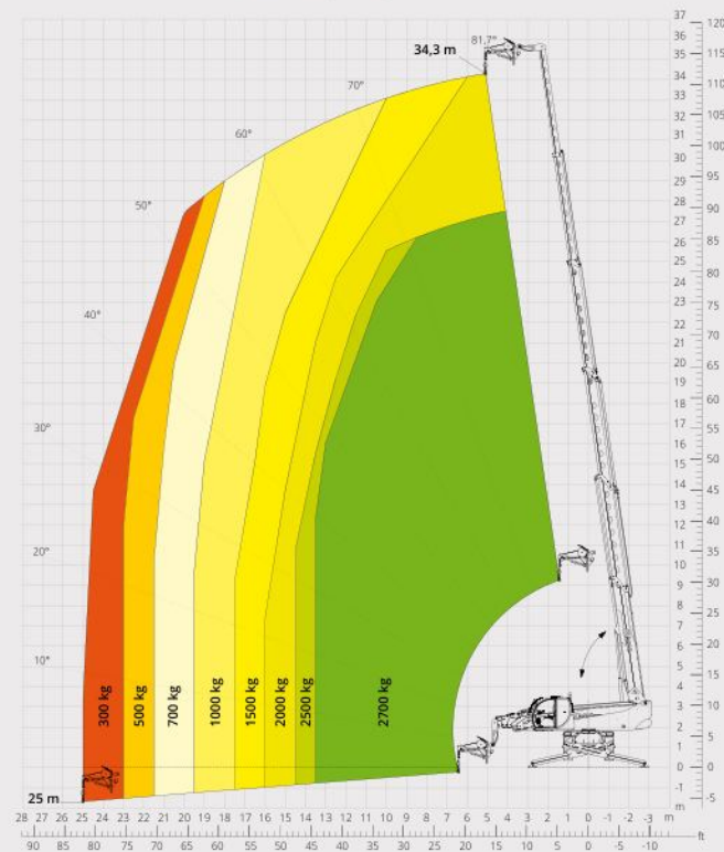
Diagram draagvermogens met GIEK MET LIER 2.700 kg
