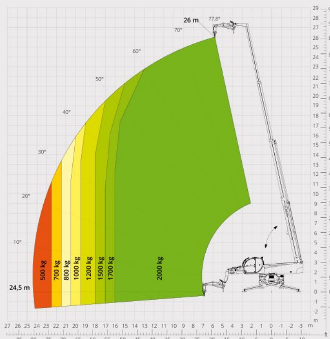
Diagram draagvermogens met GIEK MET LIER 2.000 kg ATT - 04 - 015
