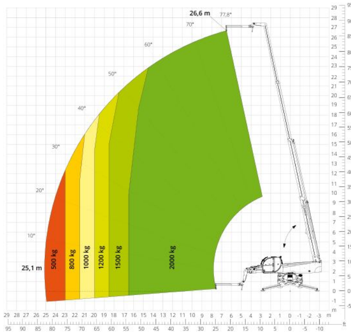
Diagram draagvermogens met ROTEREND UITKLAPBAAR WERKPLATFORM 1.000 kg ATT - 01 - 016
