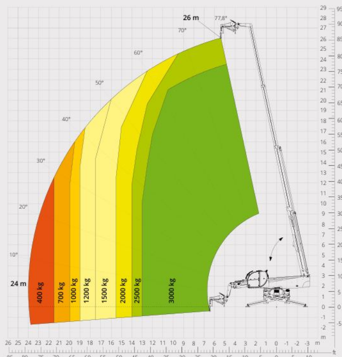
Diagram draagvermogens met GIEK MET LIER 3.000 kg ATT - 04 - 019
