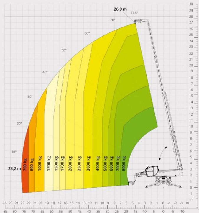
Diagram draagvermogens met HAAK 8.000 kg ATT - 05 - 003
