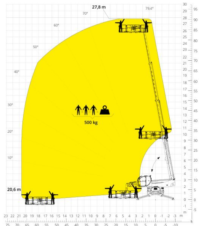
Diagram draagvermogens met ROTEREND UITKLAPBAAR WERKPLATFORM 500 kg ATT - 01 - 007
