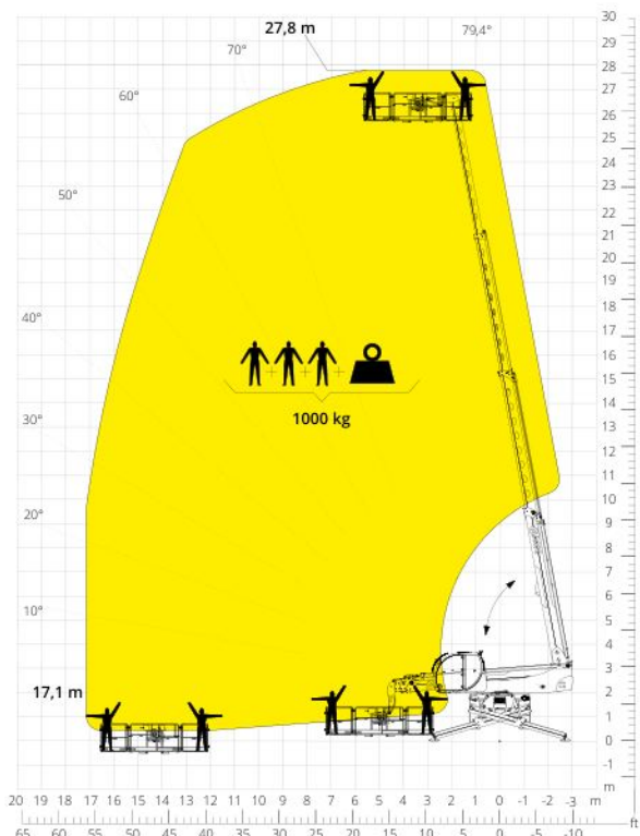
Diagram draagvermogens met ROTEREND UITKLAPBAAR WERKPLATFORM 1.000 kg ATT - 01 - 016
