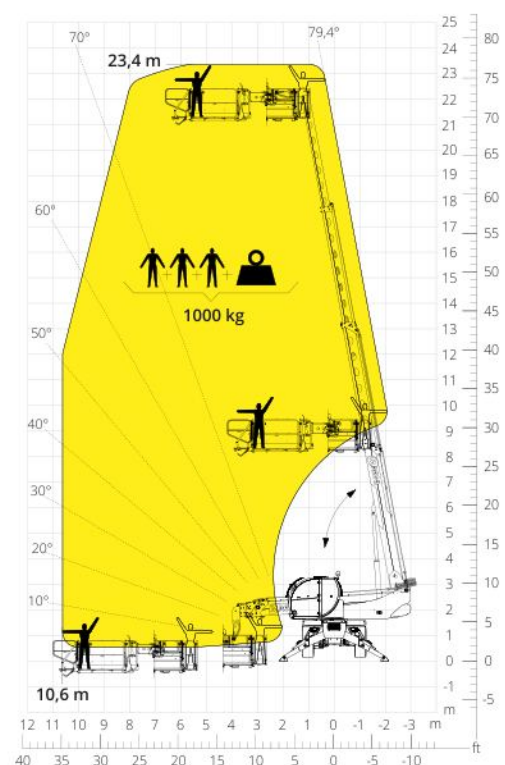
Diagram draagvermogens met UITKLAPBAAR WERKPLATFORM VOOR DAKEN 1.000 kg ATT - 01 - 020
