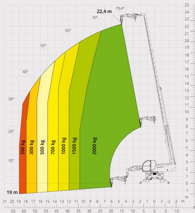
Diagram draagvermogens met GIEK MET LIER 2.000 kg
