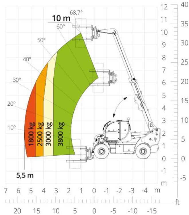
Diagram draagvermogens met BANDENKLEM 3.800 kg ATT-06-005
