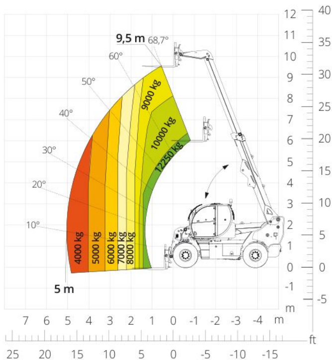
Diagram draagvermogens met VORKEN MET KLEPSTANDSTELLER 12.000 kg ATT-03-050
