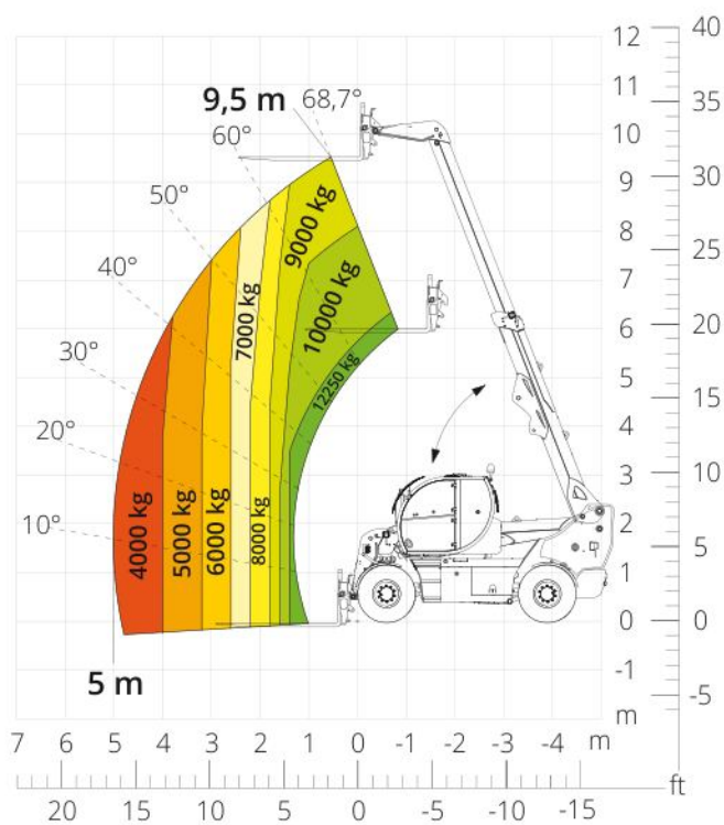
Diagram draagvermogens met VORKEN MET KLEPSTANDSTELLER 12.000 kg ATT-03-050
